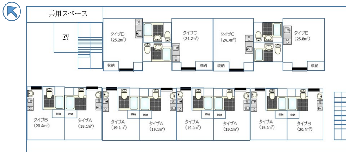
↑タイプC (24.7㎡)
